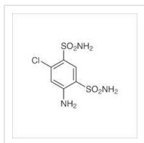
4-Amino-6-Chlorobenzene-1,3-
