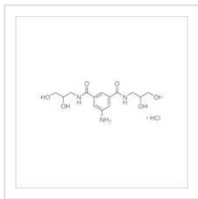
R-(-)-1-((4-Chlorophenyl)Phenyl)...
